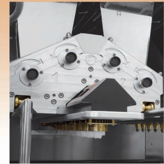
■ Corps de dosage
